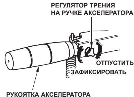
РУКОЯТКА АКСЕЛЕРАТОРА
