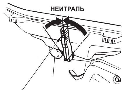
РЫЧАГ ПЕРЕКЛЮЧЕНИЯ МУФТЫ РЕВЕРСА
